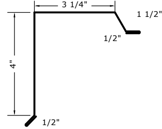
RAKE
