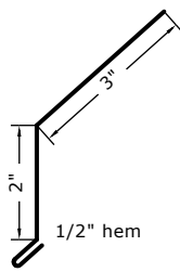
DRIP EDGE
